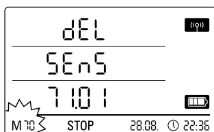
Exemple d'affichage : sélection de la fonction de déconnexion M70 pour la déconnexion du premier capteur connecté.
